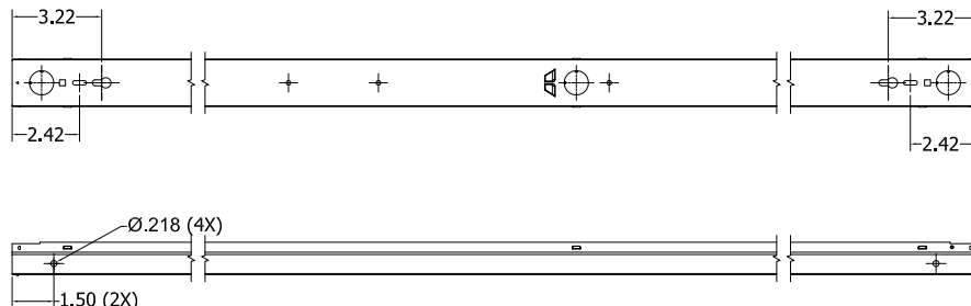
MNS5 and MNS8 Mounting Hole Dimensions
