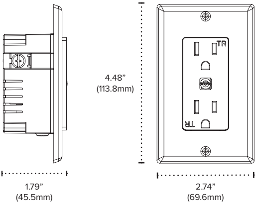
SPEKTRUM+ SMART OUTLET RECEPTACLE DIMENSIONS
