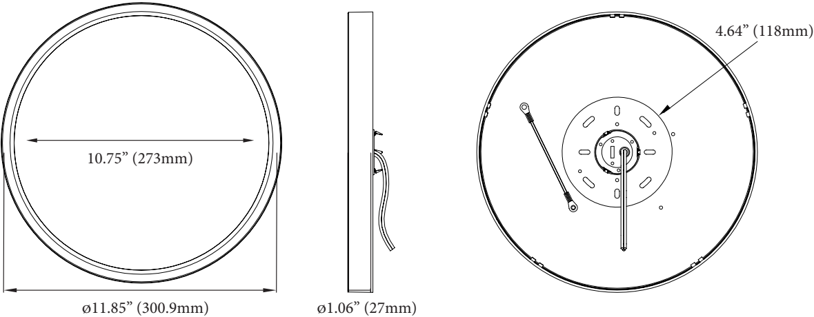
SPKPL-SF10-RGBTW-WH
