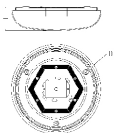
CL-A6111-6-LED02 Dimensions mm | 279(D) x 95(H) inch | 11(D) x 3.8(H)
