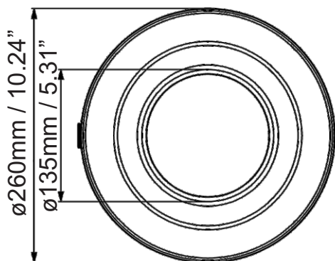
CDFP 8" - 120-347V
