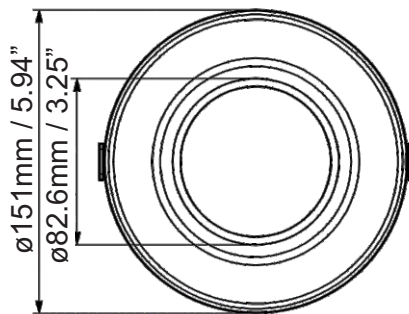
CDFP 4" - 120-347V
