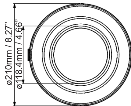
CDFP 6" - 120-347V
