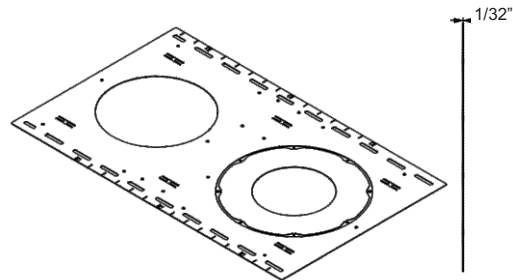
CDFP-SJPlate01
