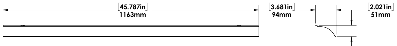
Wings dimensions
